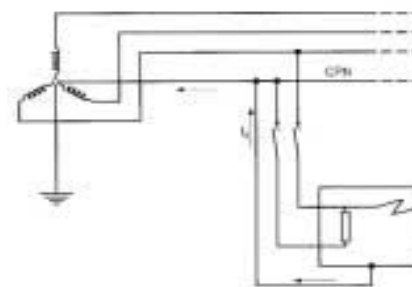
Figura 2. Esquema TN-C.
